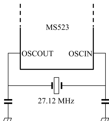
图 22. 石英晶体的连接
