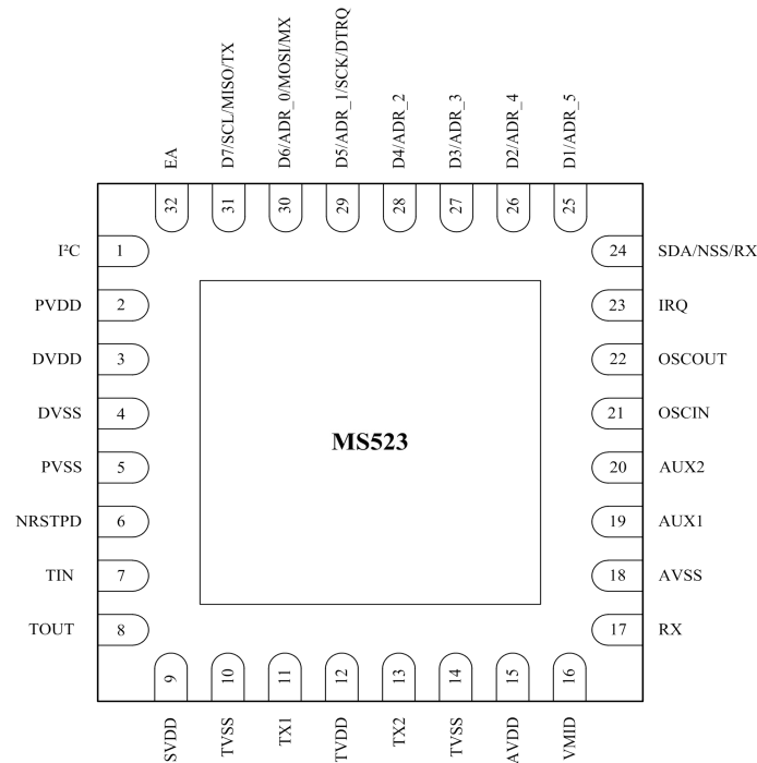
图 3. 封装
