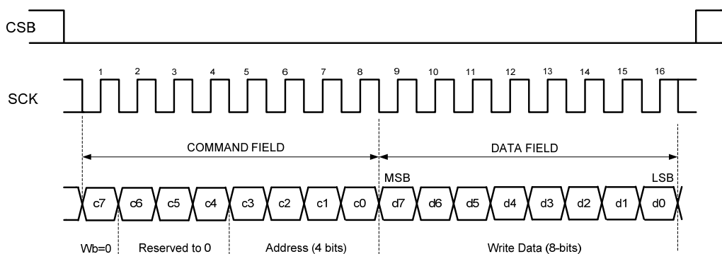
图 9 SPI 串口协议
