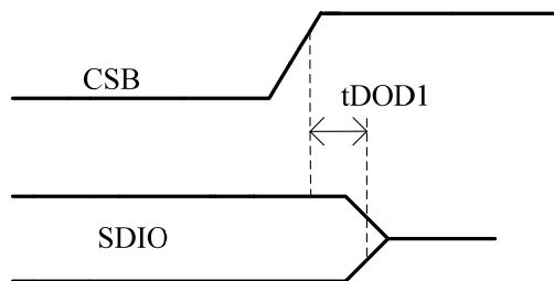
图6 CSB上升沿到来之后SDO的禁用时间
