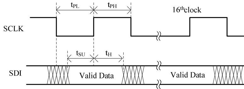
图2 SPI建立保持时间
