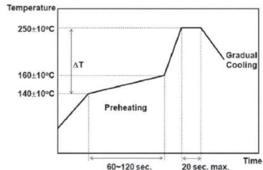
Vapor Reflow
