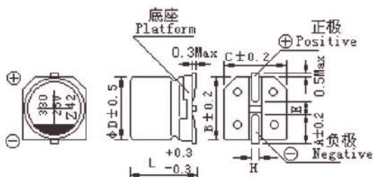
(Φ6.3 X 7.7 / Φ8 ~ Φ10 X 10.2)
