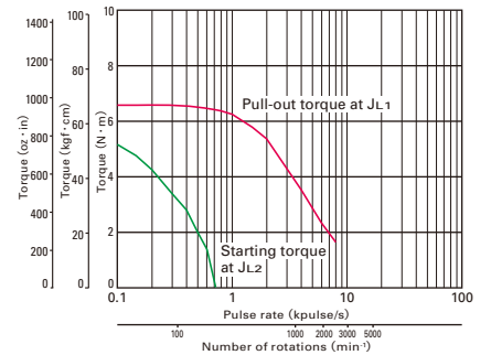
● 103H8223-63 □□
