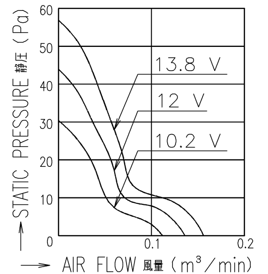
風量-静圧特性例
