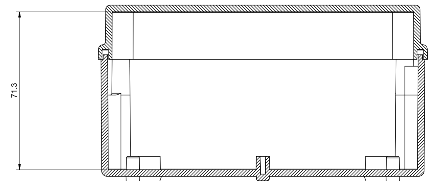
Sezione A-A
