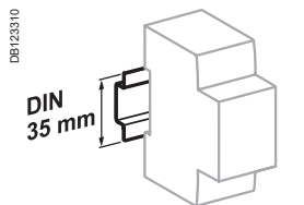
Clip on DIN rail 35 mm (1.38 in)
