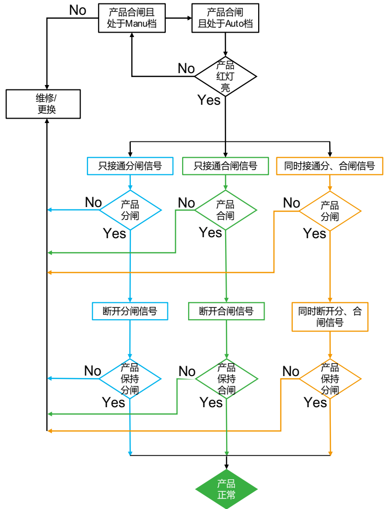
RCA逻辑图
