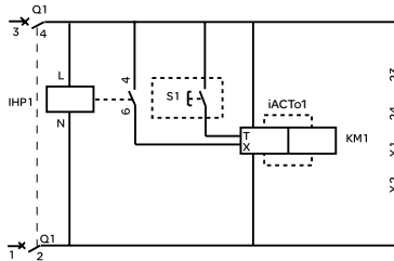
控制回路
