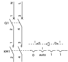
电源回路
