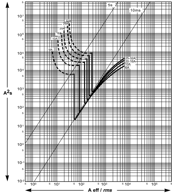
热应力曲线
