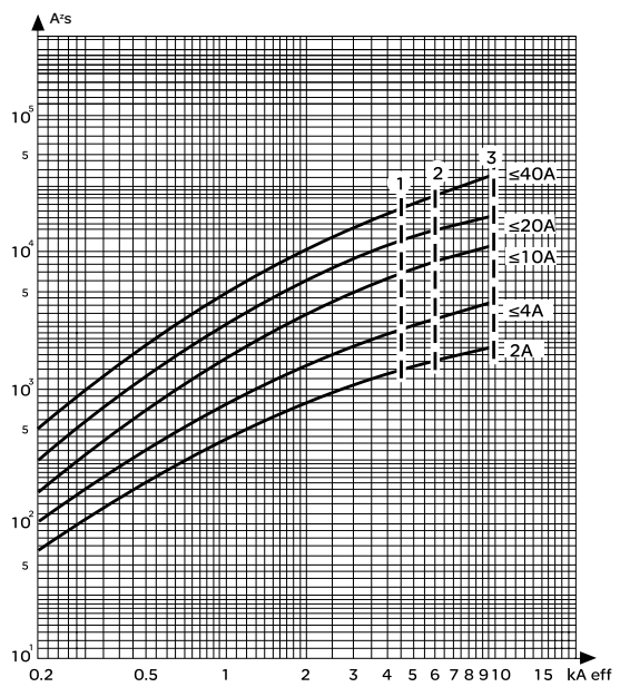
热应力曲线
