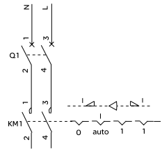
电源回路
