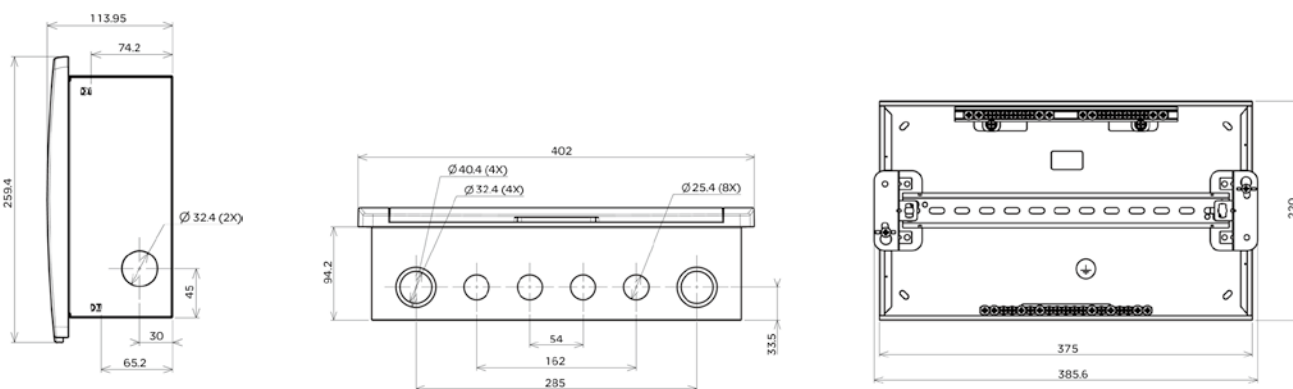
暗装箱 (16位)
