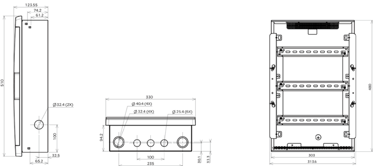
暗装箱 (36位)
