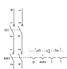
电源回路
