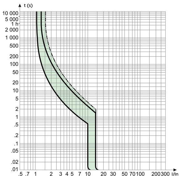
D曲线
