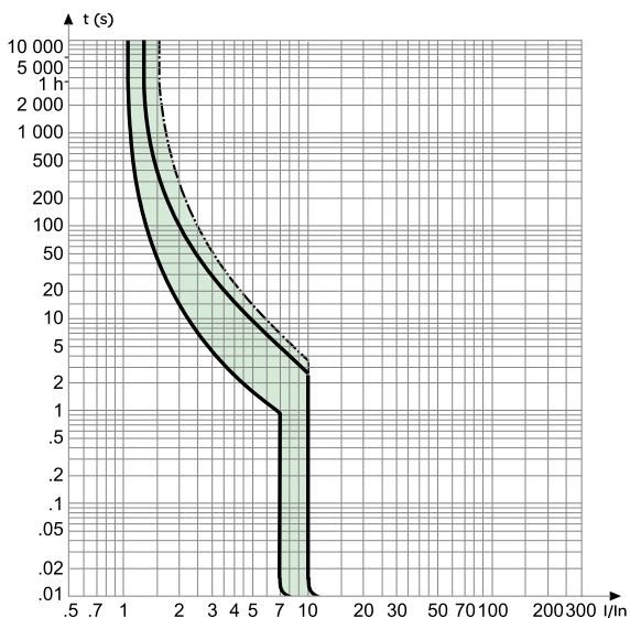
C曲线
