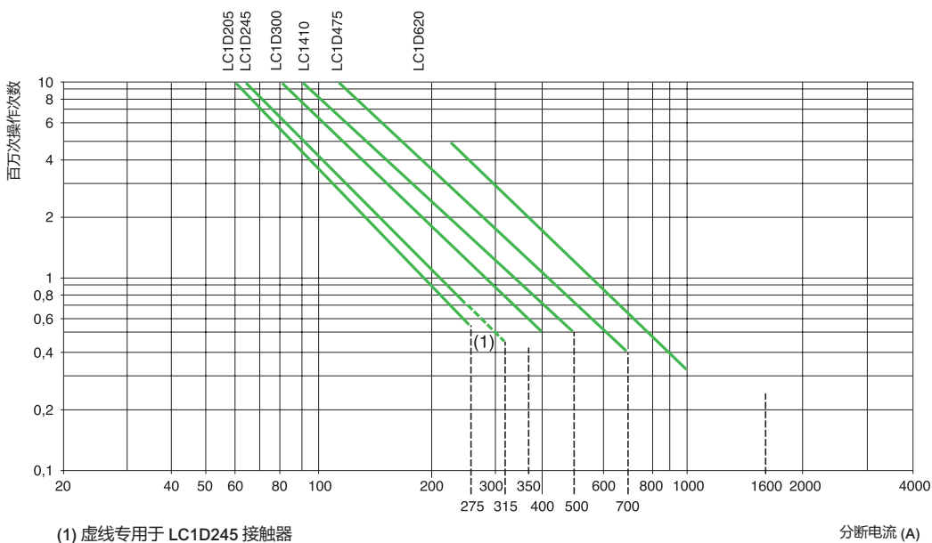
(1) 虚线专用于 LC1D245 接触器
