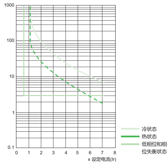
类别 30 的脱扣曲线
