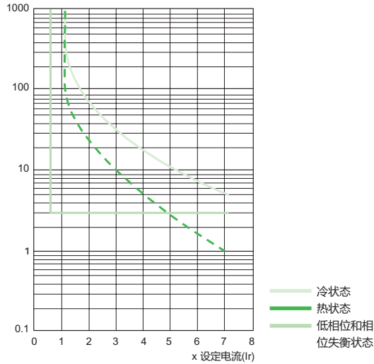
类别 20 的脱扣曲线
