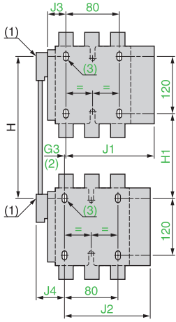
装配 A
