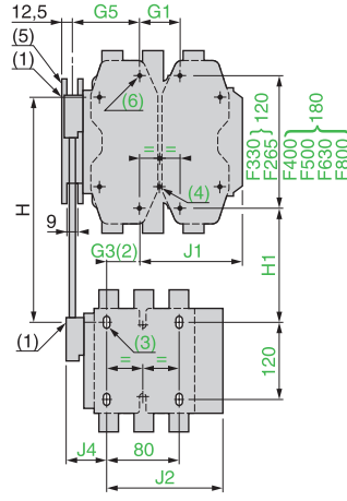
装配 B
