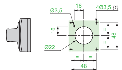
柜门钻孔
