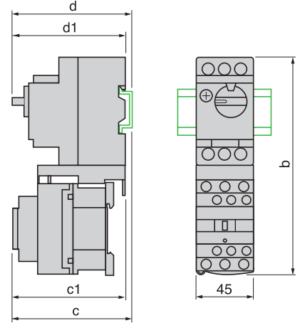
用于组合 GV2PM + D 型接触器
