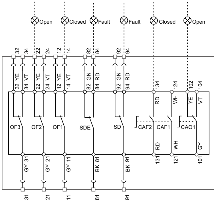
如图所示，电路已断电，所有设备均处于断开状态。○所示的端子需由客户连接。
