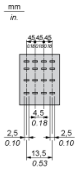
销钉侧视图
