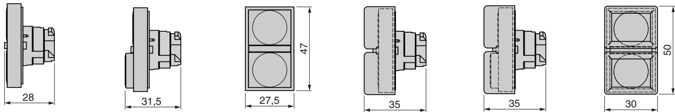
ZB4-BA81●●, ZB4-BA82●●
