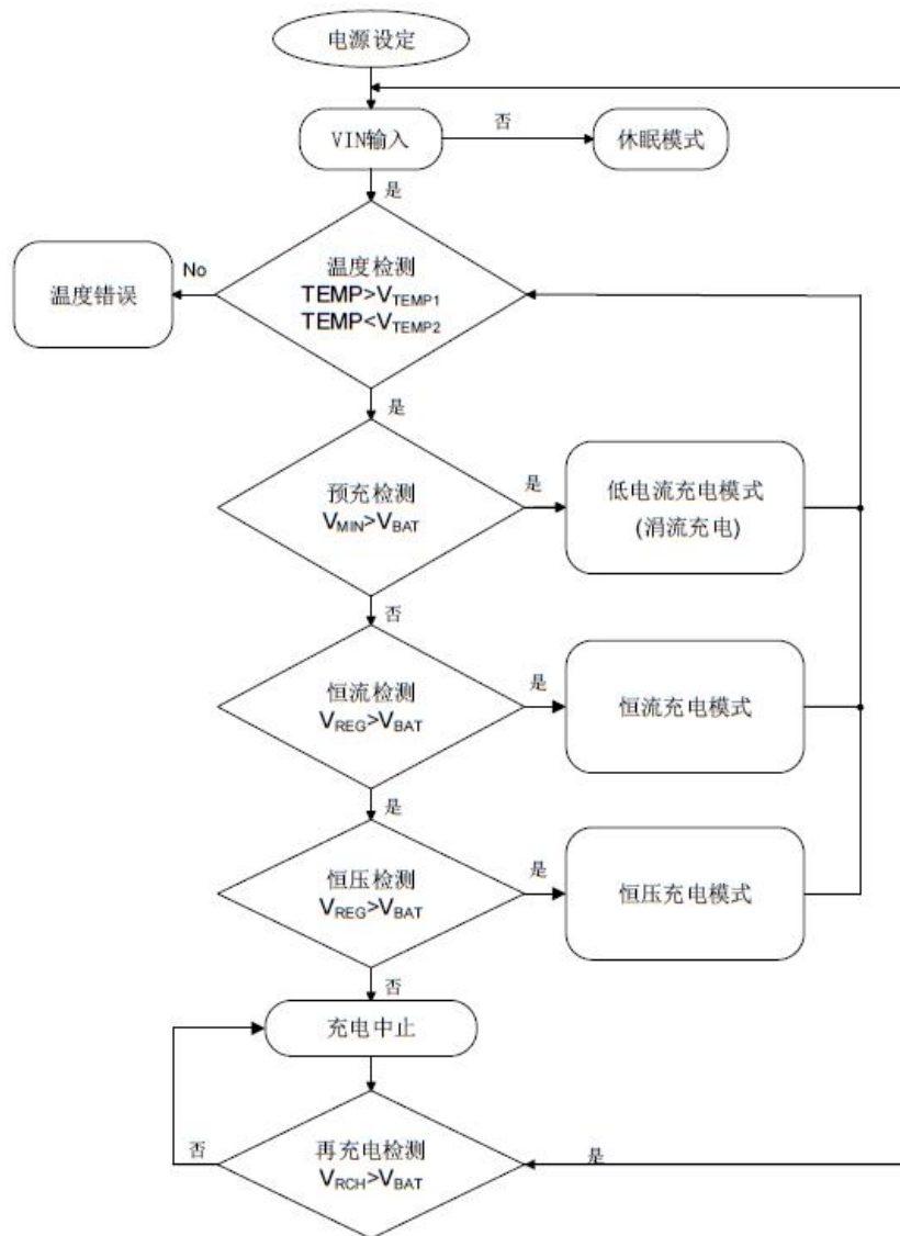
图1 工作流程图
