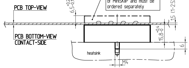
MiniSKiiP 2
