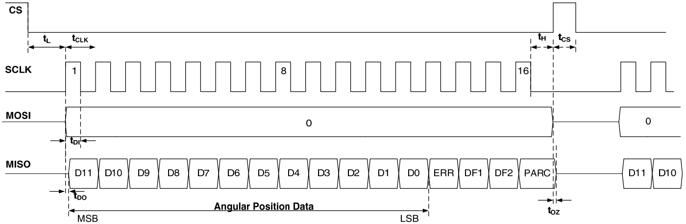
SPI 时序图
