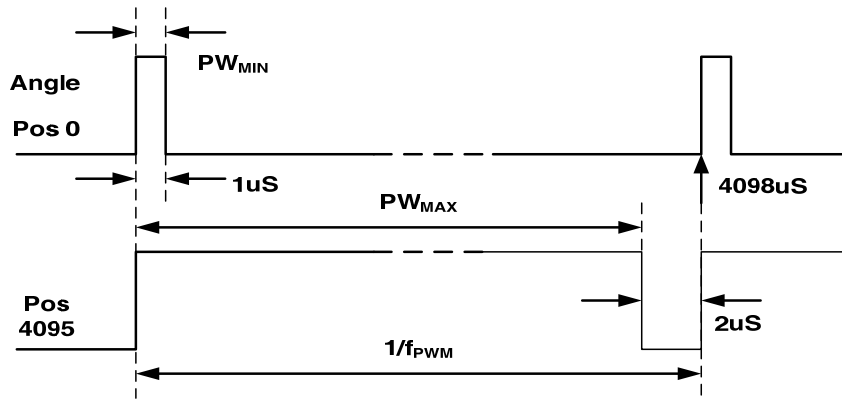
f_{\text{PWM}}=244\text{Hz} , PWM 波形示意
