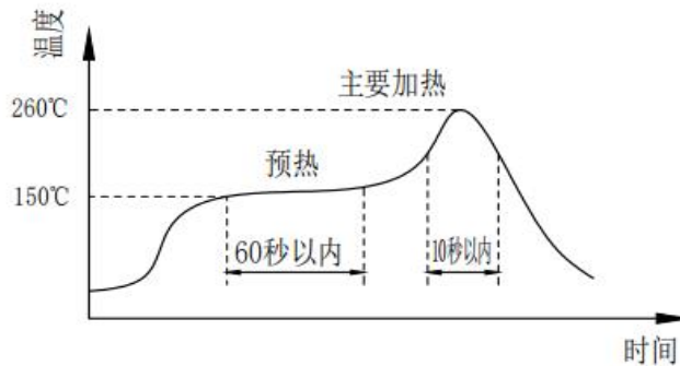
图 4.回流焊接
