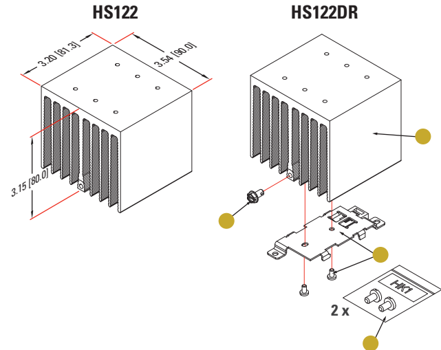
DIN Rail Bracket
