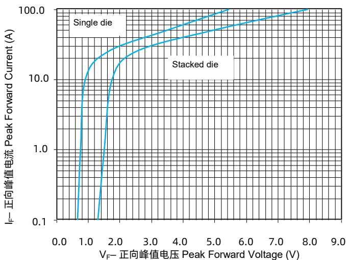
FIGURE 8 峰值正向电压及电流(典型值)
