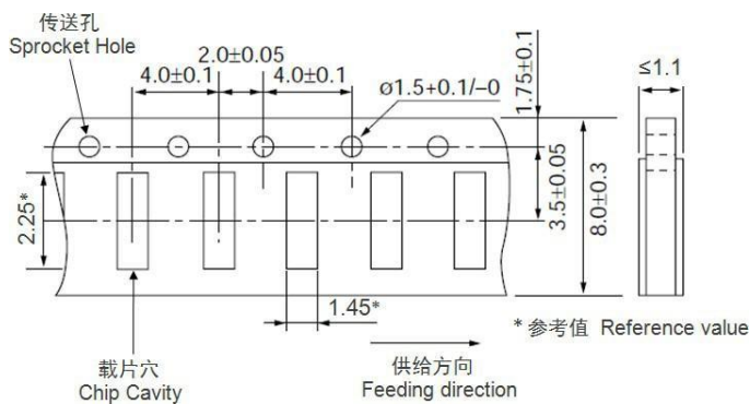
CMFB 系列 CMFB series
