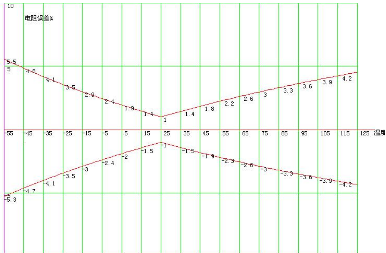
南京时恒阻值误差曲线图
