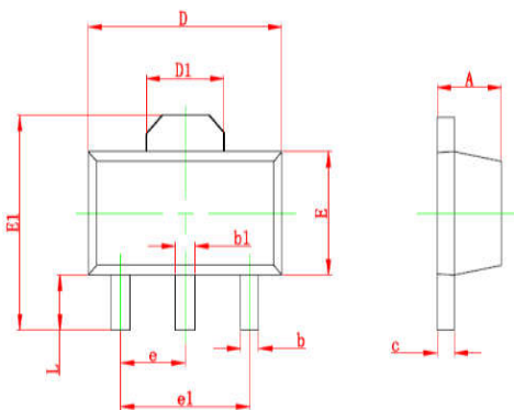
SOT-89
