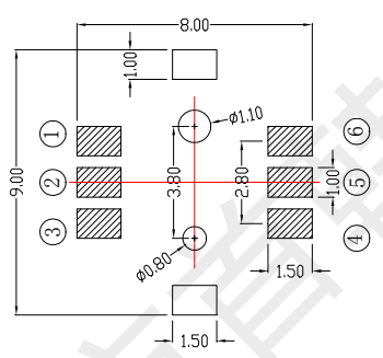
印制板安装孔图
