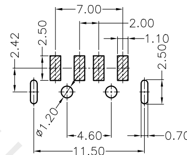
P.C.B LAYOUT(TOL:±0.05)
