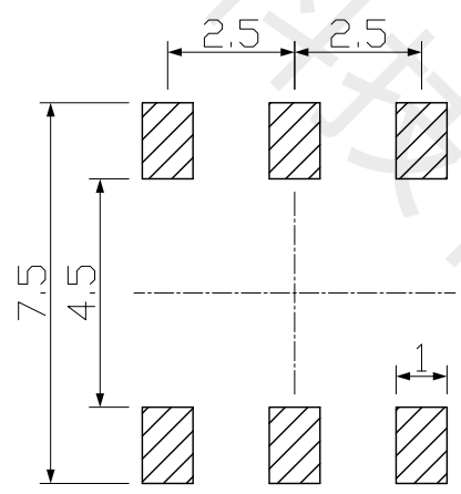
印制线路板 Recommended P.C.B layout
