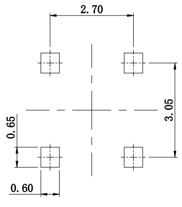
印刷板安装孔图 P.C.B Mounting pattern dimension
