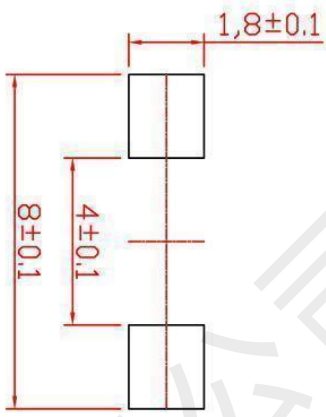
PCB. 焊接图
