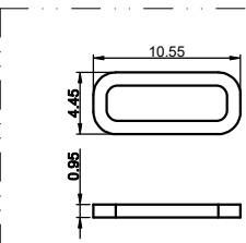
防水圈图示
