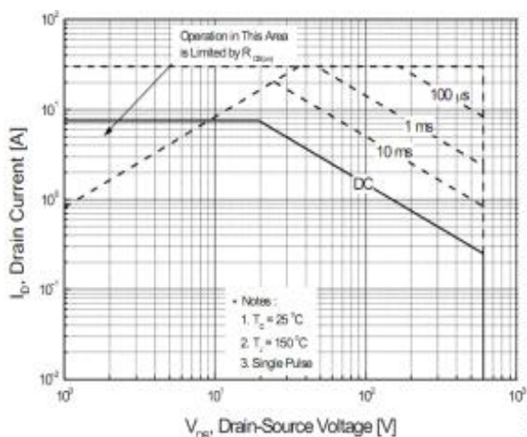
图 6-1 SIF7N60F(TO-220/262/263) 最大安全工作区曲线 Fig6-1 Maximum Safe Operating Area
