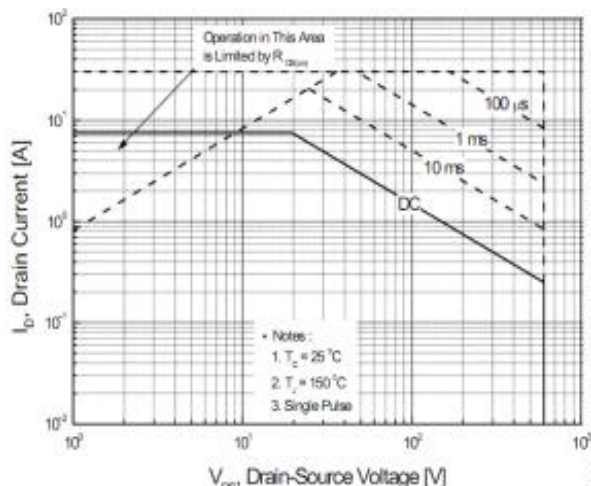
图 6-2 SIF7N60F(TO-220FP) 最大安全工作区曲线 Fig6-2 Maximum Safe Operating Area
