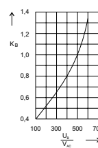
Umrechnungsfaktor für den Ausschalt i²t-Wert Reduction factor for total i²t-value
