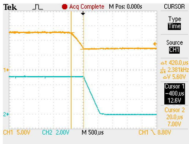
Vin=12Vdc, Po=10W, 关机 通道 1: 输入电压 5V/格 通道 2: 输出电压 2V/格
