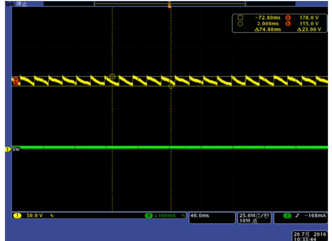
264Vac CH1:Vo
