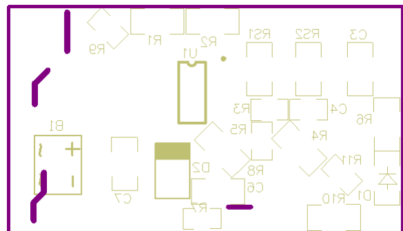
底层丝印
