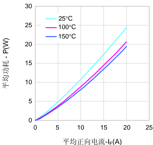
图3: 功耗（单个管脚）
