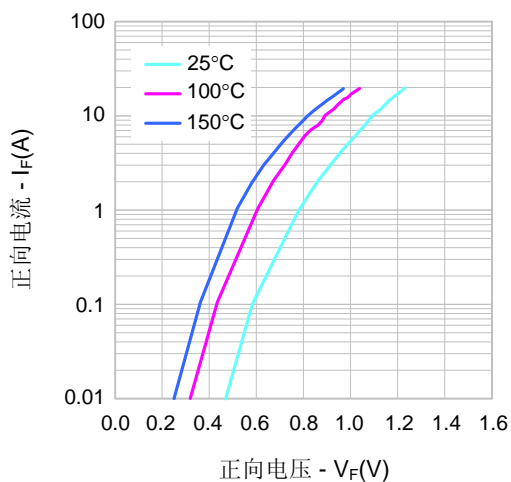
图 1: 正向特性
