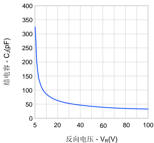
图 4: 结电容特性
