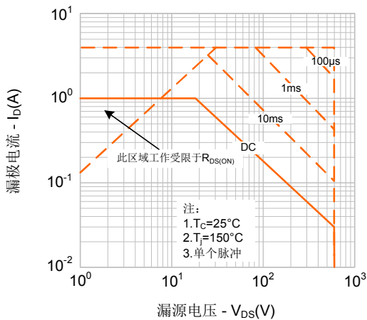
图9-3. 最大安全工作区域(SVF1N60AF)
