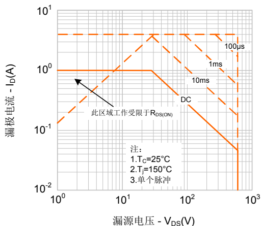
图9-1. 最大安全工作区域(SVF1N60AM/D)
