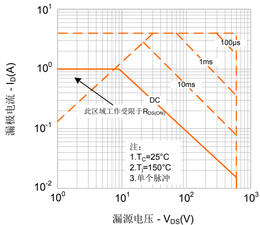
图9-2. 最大安全工作区域(SVF1N60AB)
