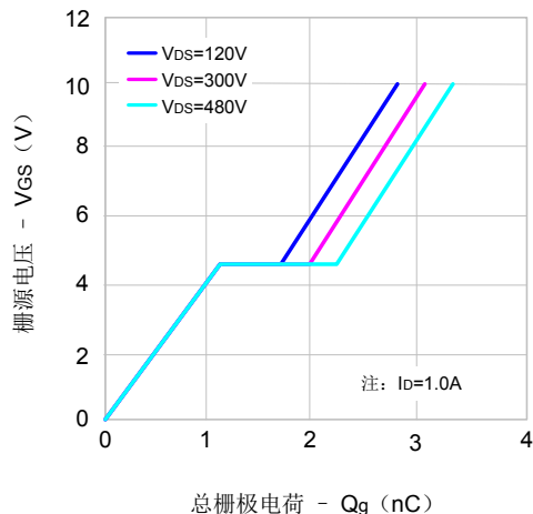
图6. 电荷量特性
