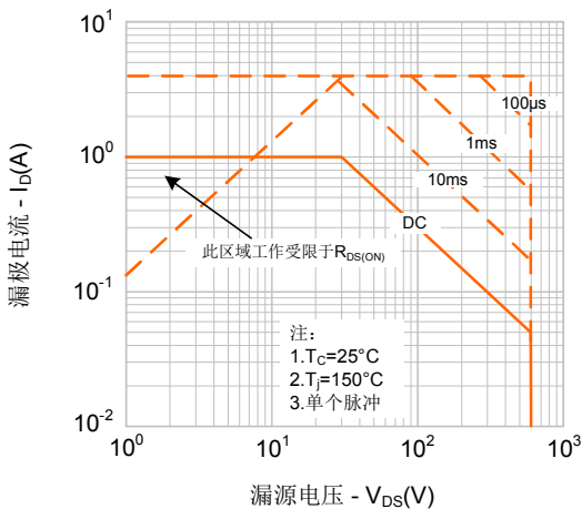
图9-5. 最大安全工作区域(SVF1N60AMJ)
