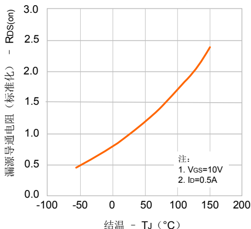
图8. 导通电阻vs.温度特性
