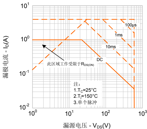
图9-4. 最大安全工作区域(SVF1N60AH)
