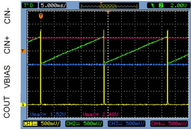
TS1108-20 Coulomb Counting V_{SENSE}=10\text{mV} , V_{BIAS}=1.5\text{V} , V_{CIN-}=2.5\text{V}
