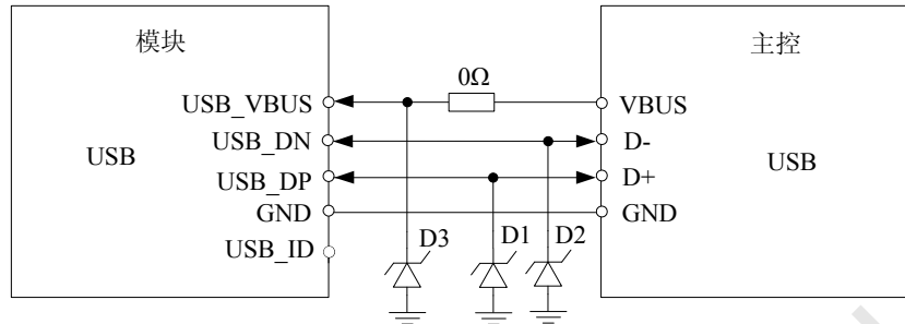
图 18: USB 连接图
