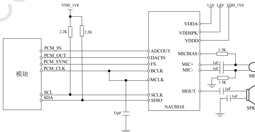
图 25: PCM 推荐电路
