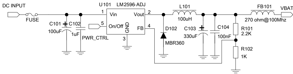
图 8：开关电源推荐电路
