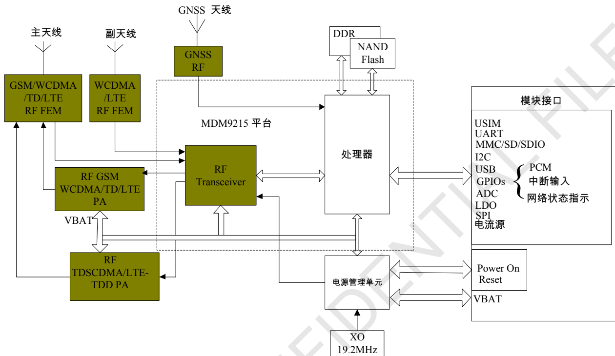
图 1：模块框图
