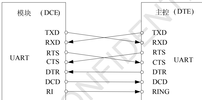
图 13: 串口连接图 (FULL 模式)
