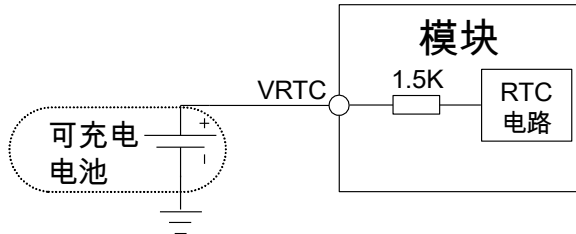
图 19: 可充电电池给 RTC 供电
