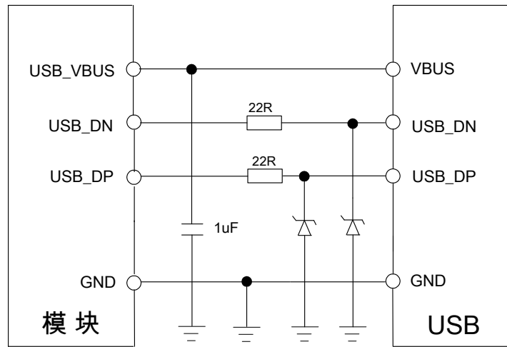
图 25: USB 连接图
