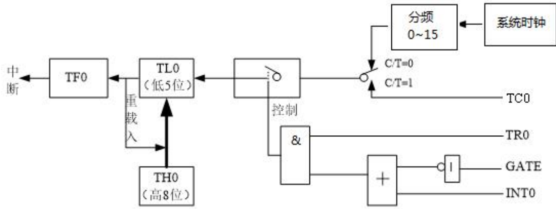
图11-4 T0/T1 方式2结构
