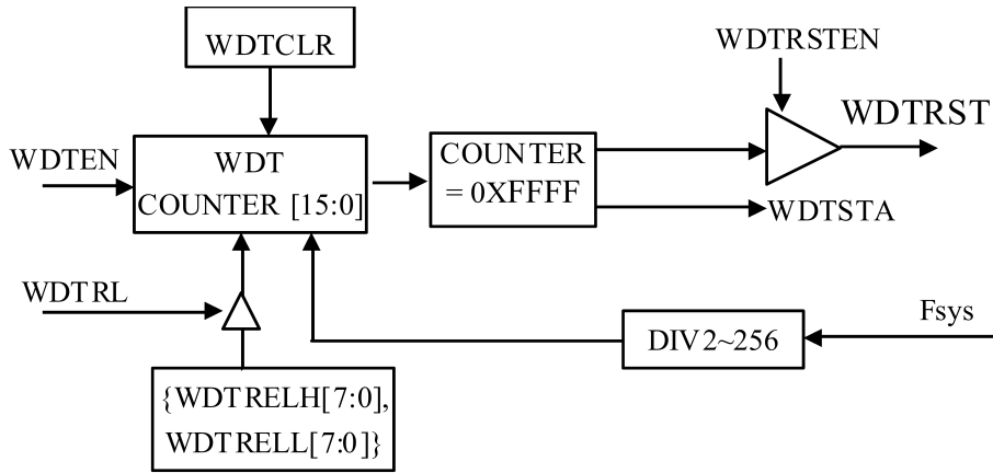
图 8-4 ASM87L164 看门狗电路模块图
