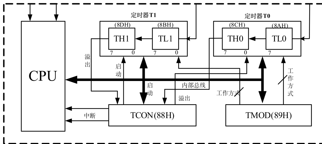
图 11-1 ASM87L164 定时器/计数器功能框图
