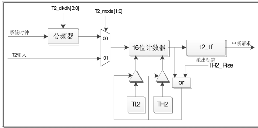
图 2 定时器 2 的定时/计数模式功能框图
