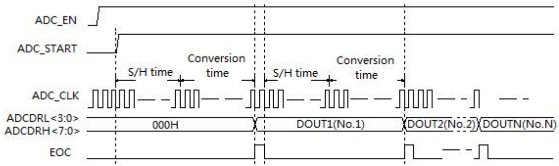
图 19-2ASM87L164ADC 转换时序图
