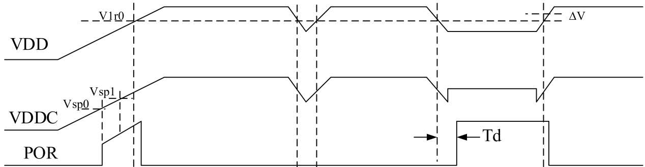
图 8-3 ASM87L164 上电复位时序示意图
