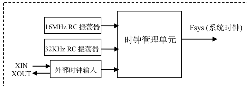
图 8-1 ASM87L164 的双时钟模式结构框图
