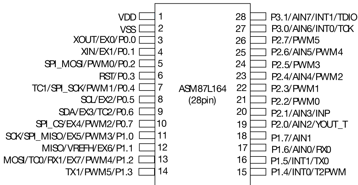
图 3-1 ASM87L164 管脚排列图 (TSSOP28 Pin)
