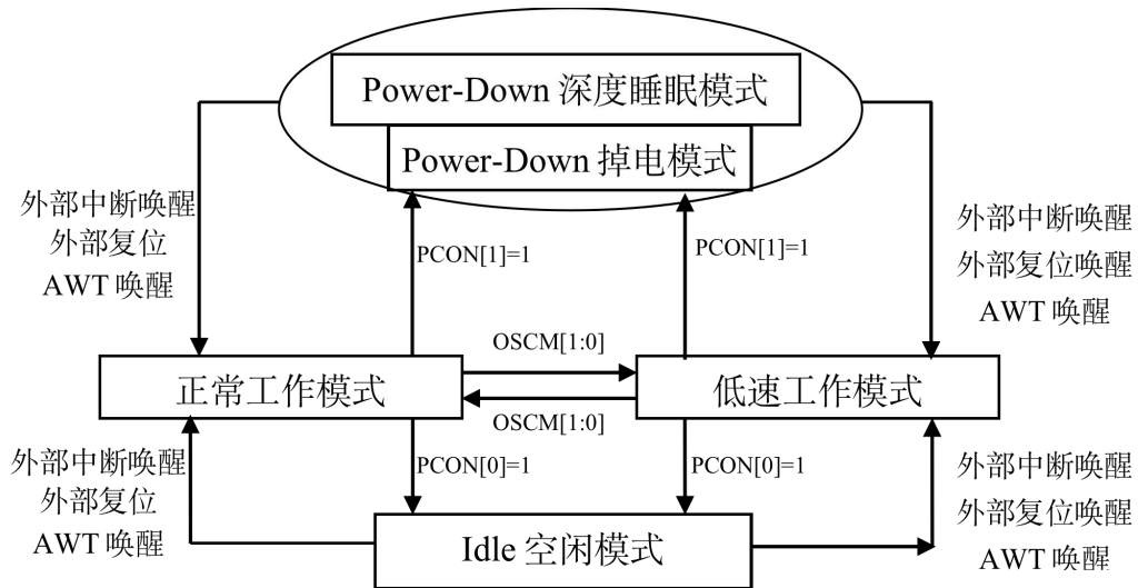
图 9-1 ASM87L164 工作模式转换示意图
