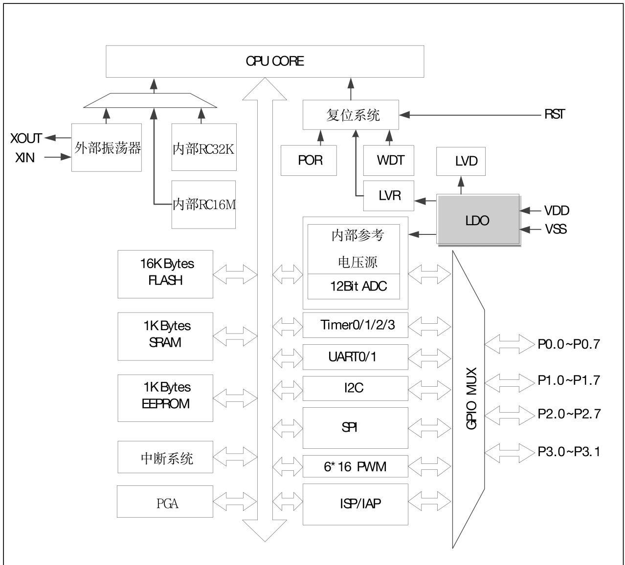
图 4-1 ASM87L164 内部功能框图
