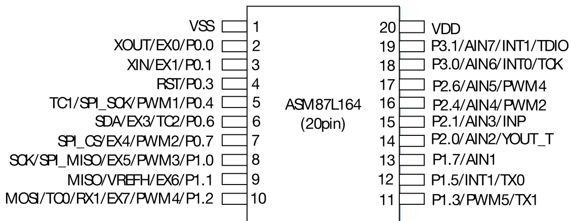
图 3-2 ASM87L164 管脚排列图 (TSSOP20 Pin)
