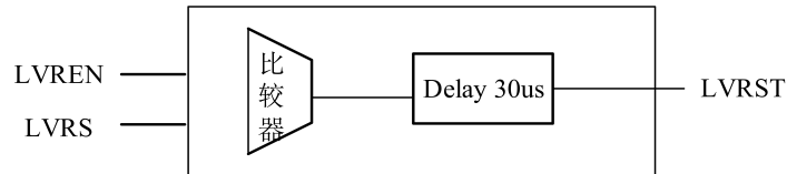
图 8-4 ASM87L164 低电压复位模块图
