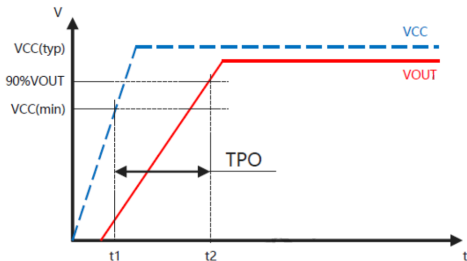
图 1：上电时间定义
