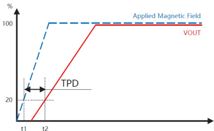
图 2：传输延迟定义
