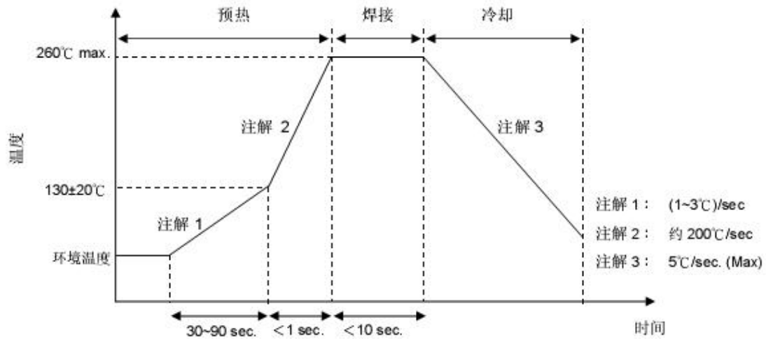
波峰焊曲线
