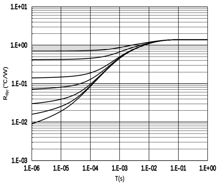
图 7 瞬态热阻抗
