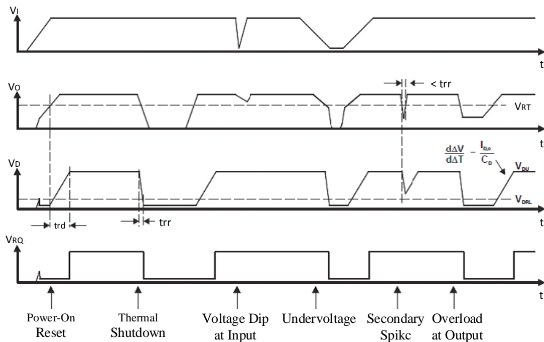
6-1 复位时序
